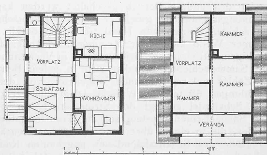
Abb. 2. Grundrisse vom Erdgeschoss und Dachstock zu Abb. 1. Massstab 1:250.
