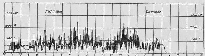
Abb. 69. Belastungs-Diagramm «Unruhig» vom 21. Januar 1908. Maximale Belastung 1280 kw. — Anzahl kw./Std. 5600. Die strichpunktierte Horizontale stellt die auf 19\frac{1}{2} Std. verteilte mittlere Belastung = 287 kw. dar.
