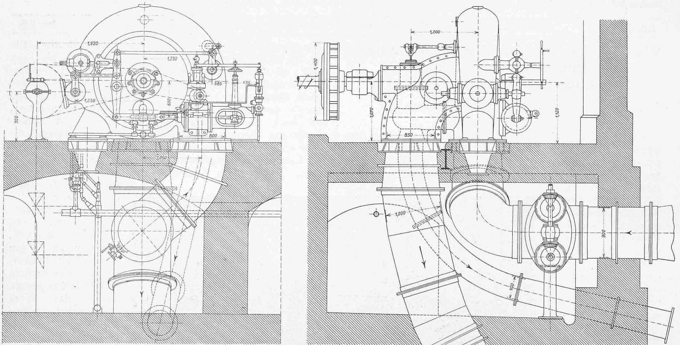
Abb. 64. Vorderansicht, Seitenansicht und Grundriss der 1300 PS-Spiral-Francis-Turbine von Escher Wyss & Cie. — Masstab 1:60.
