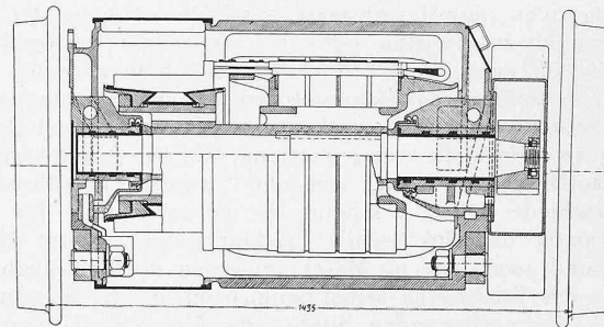
Abb. 5. Gleichstromvorgelegemotor der Westinghouse Co. für die Untergrundbahn New-York. — 1 : 20.
