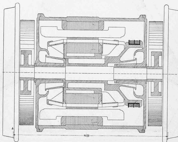
Abb. 7. Drehstromvorgelegemotor für die Siemens-Schnellbahnlokomotive Berlin-Zossen. — 1:20.
