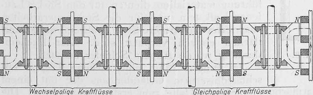
Abb. 14. Variante der Anordnung nach Abb. 13 für Doppelmotoren mit achsial verlaufendem, wechsellipoligem oder gleichpoligem magnetischem Kraftfluss zum Betrieb mit Gleichstrom oder Einphasenwechselstrom. Masstab 1 : 50.
