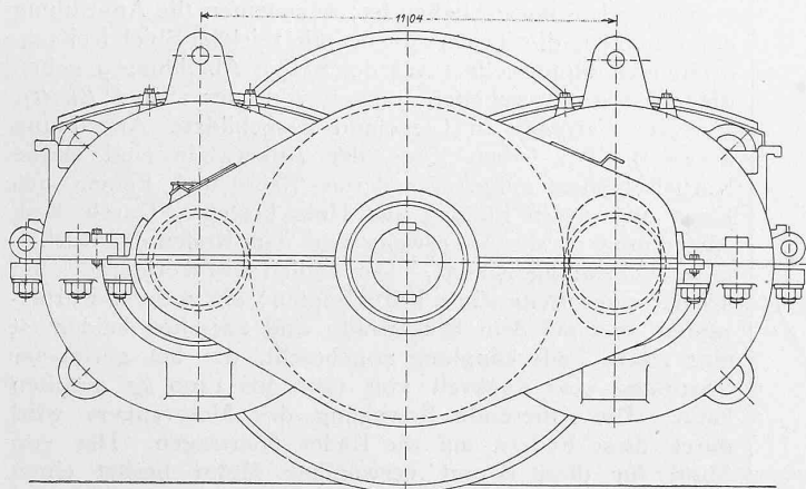
Abb. 6. Vorgelegedoppelmotor für Gleichstrom nach Křizik. — 1:20.
