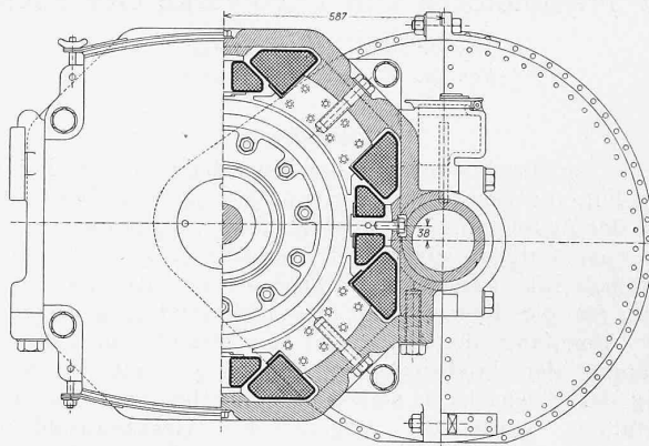
Abb. 3. Gleichstromvorgelegemotor der Siemens-Schuckertwerke für Schmalspurbahnlokomotiven. — 1 : 20.
