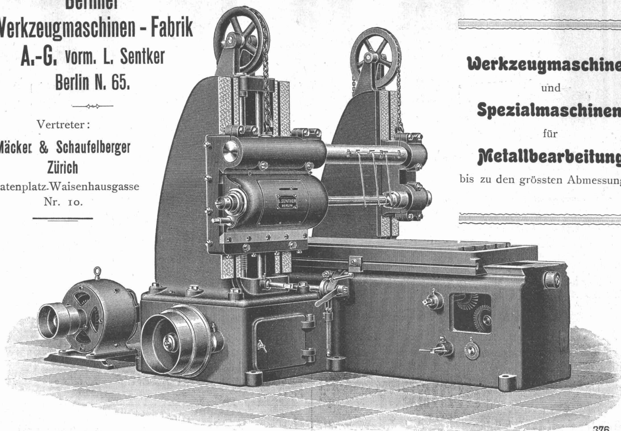
Langfraismaschine.
