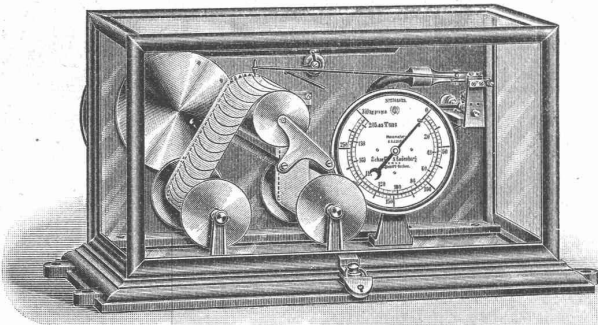
Manometer mit Aufzeichnung.
