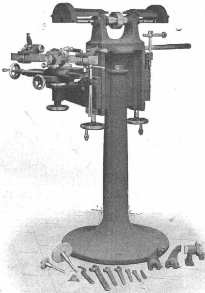
Werkzeugschleifmaschine.
