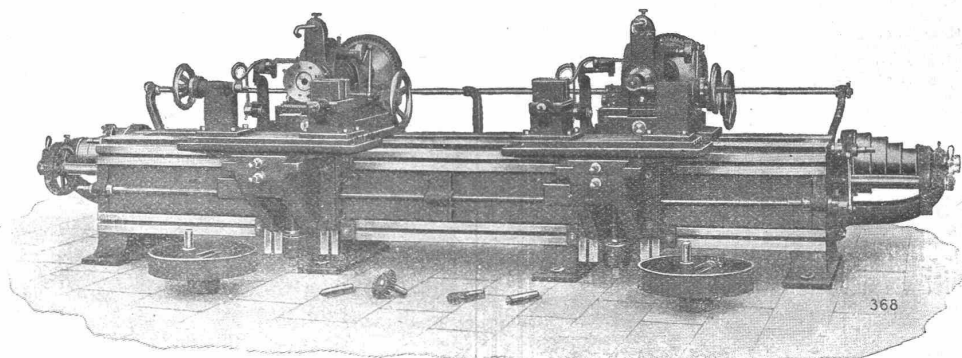
Doppelte Pleuelstangen-Bohr- und Fräsmaschine.
