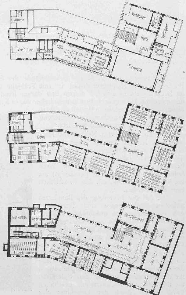
Abb. 3 bis 6. Grundrisse vom Untergeschoss, Erdgeschoss und Garten, Obergeschoss und Dachgeschoss. — Massstab 1:800.
