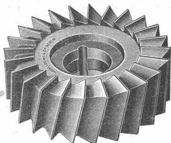
Walzenstirnfräser.
