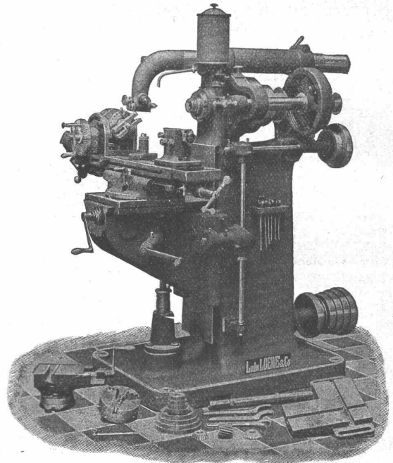
Universalfräsmaschine.
