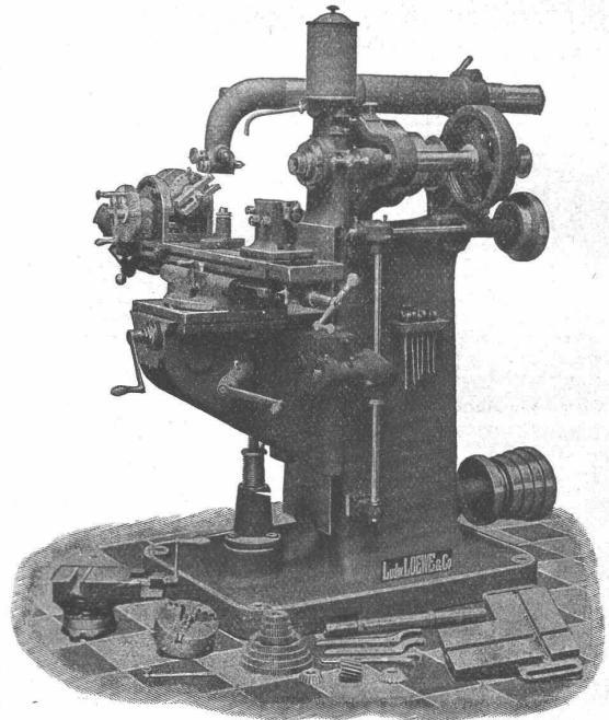
Universalfräsmaschine.
