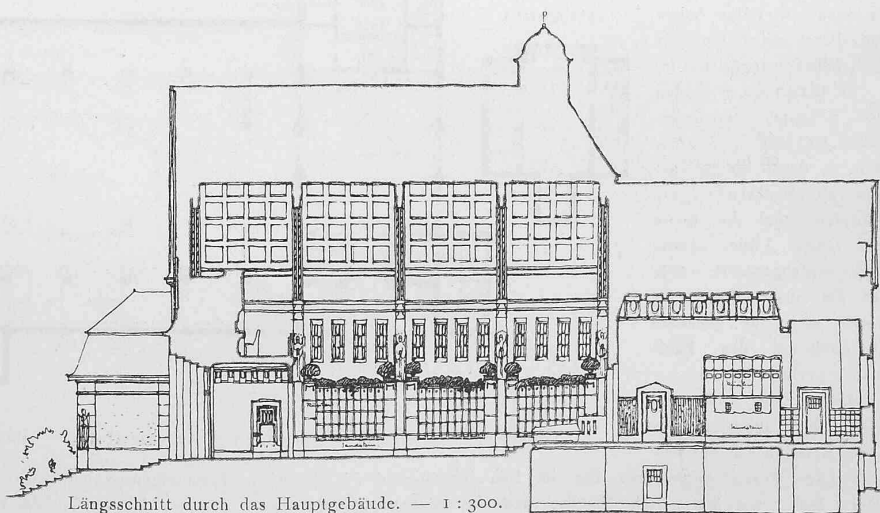
Längsschnitt durch das Hauptgebäude. — 1 : 300.
