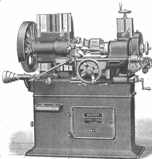
Rundfräsmaschine.
