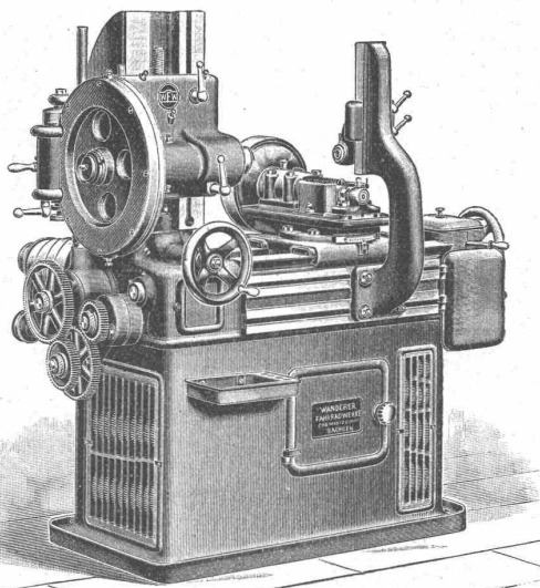
Automat. Stirnrad-Fräsmaschine.
