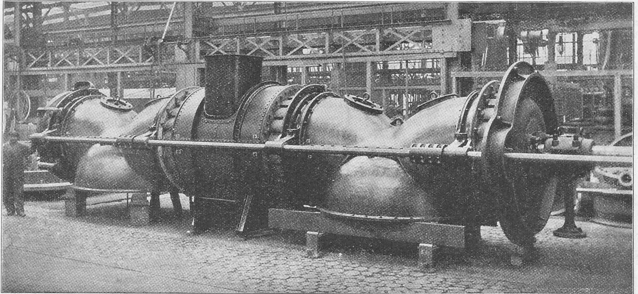
Abb. 9. Ansicht einer ganzen Turbinengruppe.
