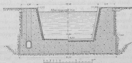
Abb. 10. Querschnitte der Eintrittskammer des Docks Nr. 2. — 1 : 500.
