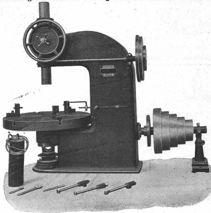
Horizontal-Bohr- und Fräsmaschine mit elektrischem Antrieb.
