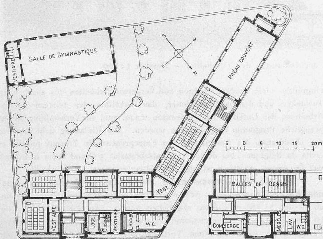
Grundrisse vom Erdgeschoss und dritten Obergeschoss. — 1 : 1000.
