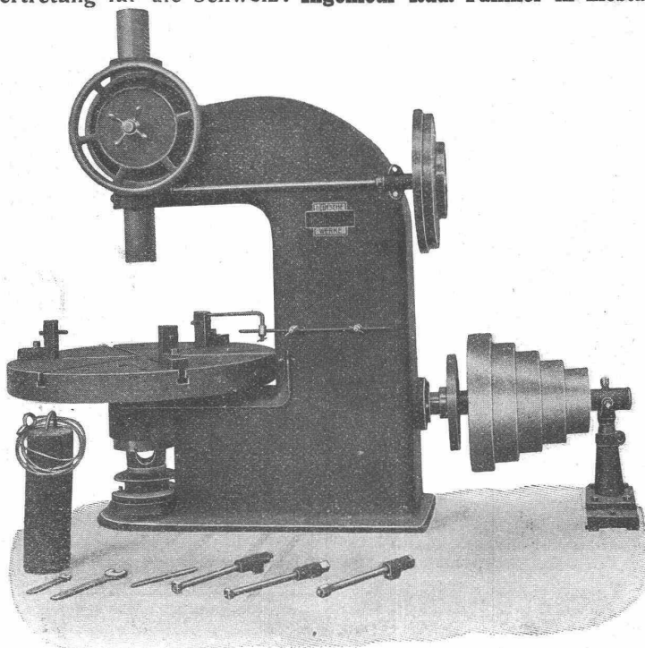
Riemenscheiben-Ausbohrmaschine.
