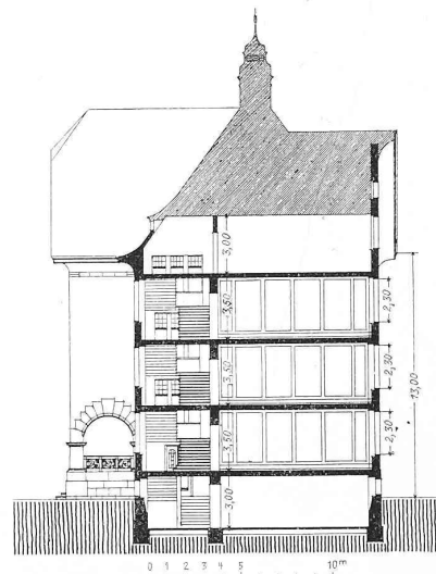
Querschnitt. — Masstab 1 : 400.
