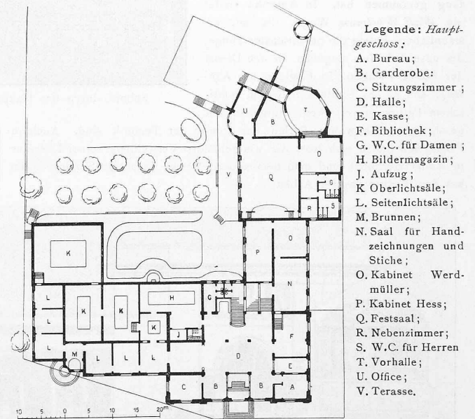
Grundrisse vom Untergeschoss und vom Obergeschoss. — Masstab 1:1000. — Grundriss vom Hauptgeschoss.
