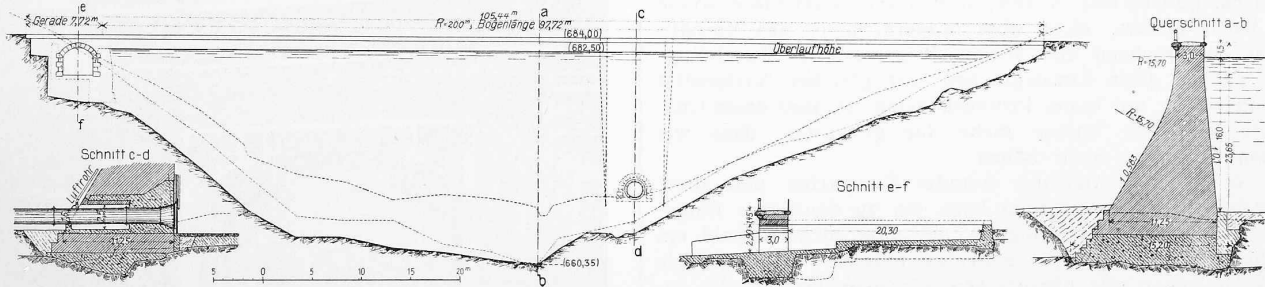
Abb. 15. Oestliche Abschlussmauer des Weihers. — Längsschnitt und Querschnitte. — Masstab 1:700.
