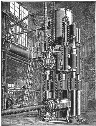
Dampfhdraulische Schmiedepresse.
