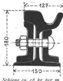
Spezial-Profil für Normalspur-Wagen.
