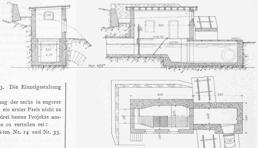
Abb. 13. Grundriss, Quer- und Längsschnitt vom Wasserschloss. Masstab 1:250.
