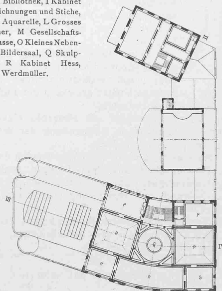
Grundriss vom I. Stock.
