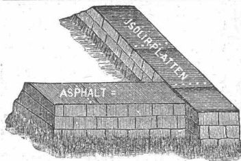
ABDECKUNG VON FUNDAMENTEN.
