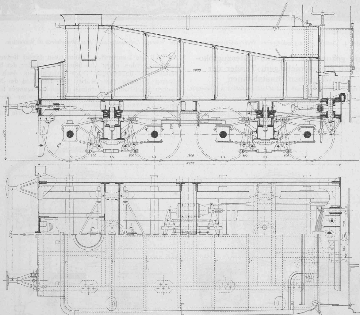
Abb. 4. Aufriss, Grundriss und Längsschnitte des Tenders. — Masstab 1 : 40.
