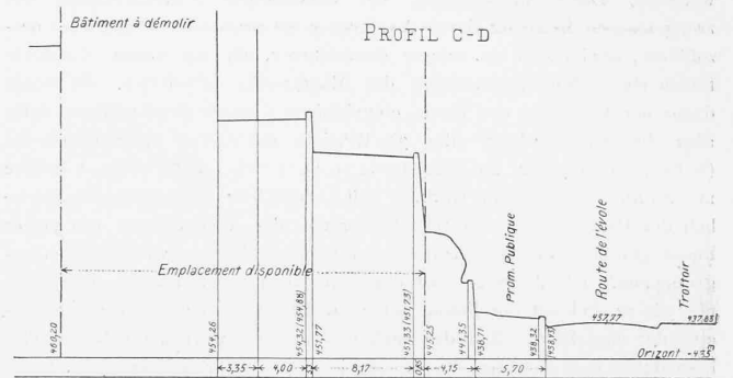
Querprofile. — Masstab 1 : 600.
