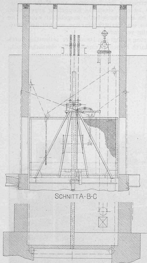
Abb. 3. Aufzug für schwere Lasten.
