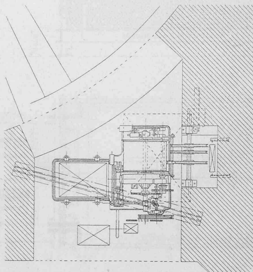
Abb. 5. Winde zum Personen-Aufzug im Justizpalast zu München.
