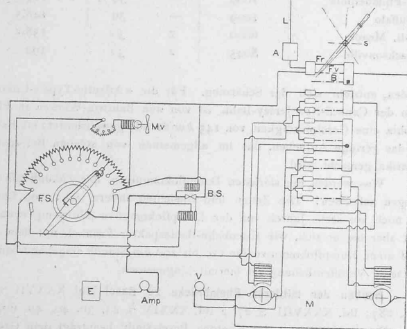
Abb. 12. Aigle-Leysin-Bahn.
