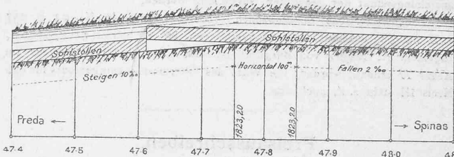
Nord. Längenprofil der Durchschlagstelle. Süd.
