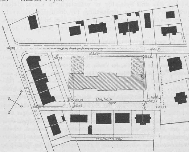
Lageplan. 1 : 2500.
