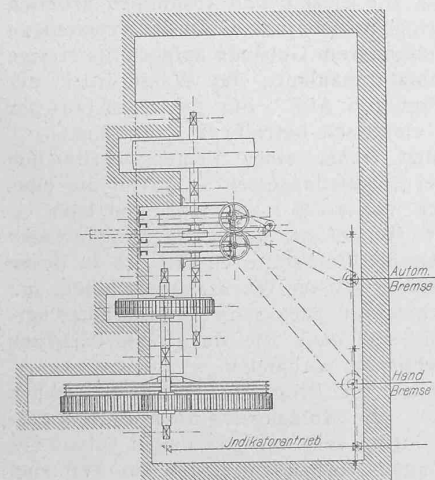
Abb. 10. Schnitt C-D. — Masstab 1:100.
