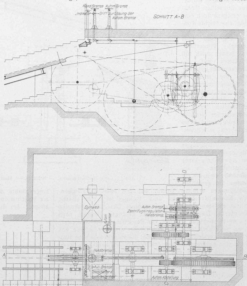
Abb. 9. Die mechanische Einrichtung auf der obren Station. — Masstab 1:100.
