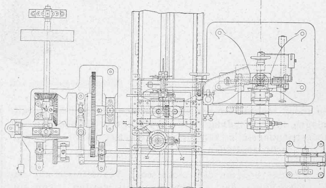
Abb. 14. Vertikale Bandsäge von Th. Bell & Cie. A.-G. in Kriens. Masstab 1:40.
