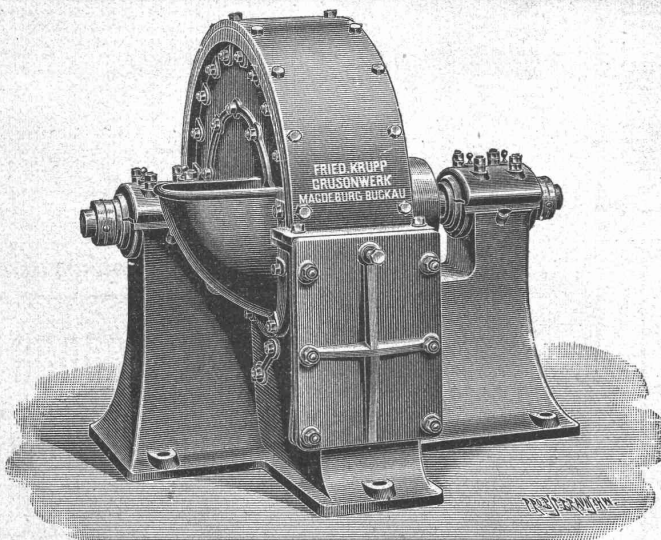
Schlagkreuzmühle.
