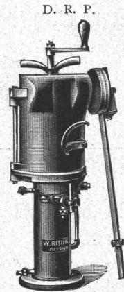
1-Stempel-Pressen.
