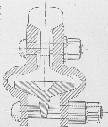
Querschnitt. — Masstab 1:3.
