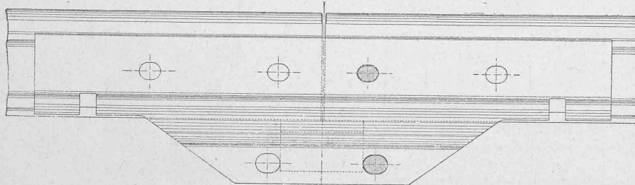
Aufriss. — Masstab 1:6.
