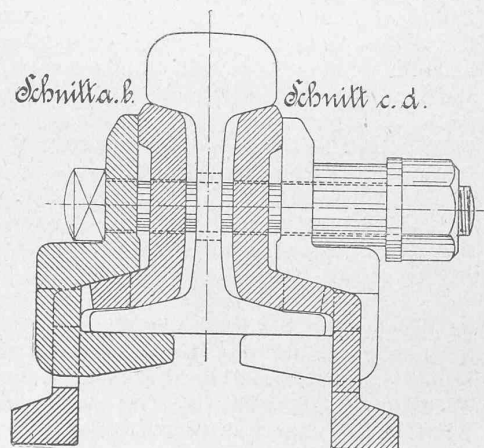
Querschnitt. — Masstab 1:3.
