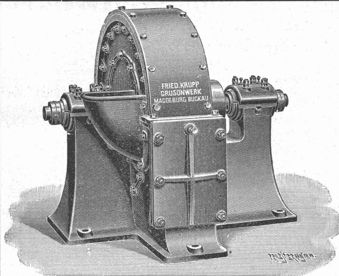
Schlagkreuzmühle.
