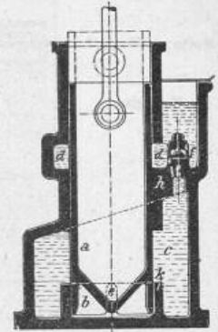
Fig. 34. Vakuumpuffer mit Oelbremse 1:8.
