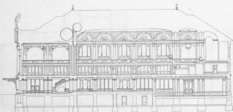
Längenschnitt 1:500.
