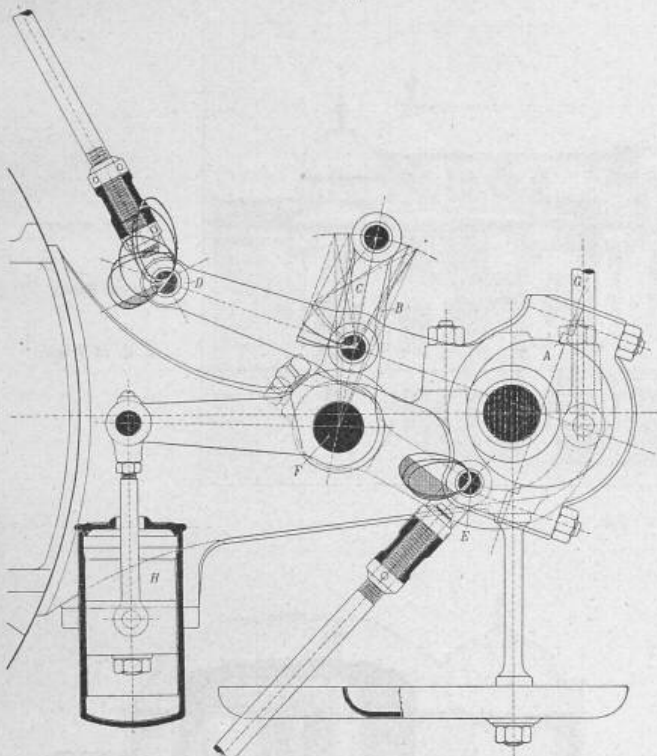
Fig. 31. Ventil-Steuerung 1:6.
