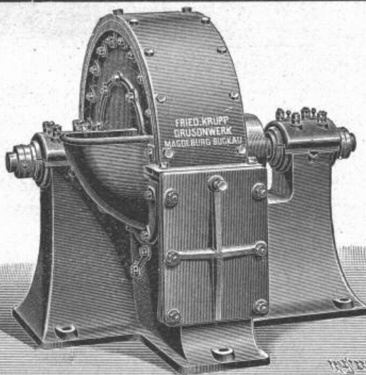
Schlagkreuzmühle.
