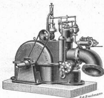
Francis-, Patent-Conus- und Centrifugal-Turbinen für Gefälle von ca. 0,3—100 Meter
