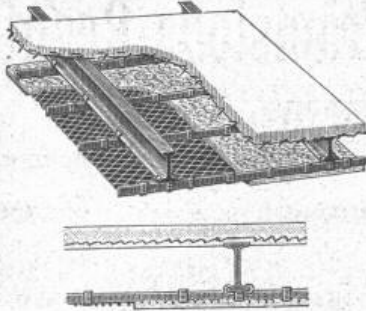
Deckenkonstruktion Hardis und Gipsplatten.
