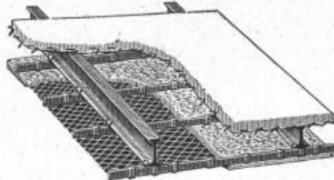
Deckenkonstruktion Hurdslatten. Gipsplatten.
