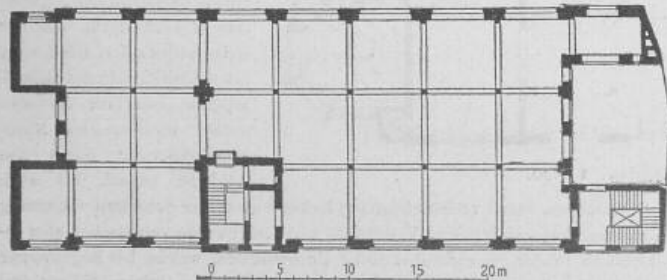
B. A. W. Fig. 75. Kaufhaus Riemer — Grundriss 1:500.
