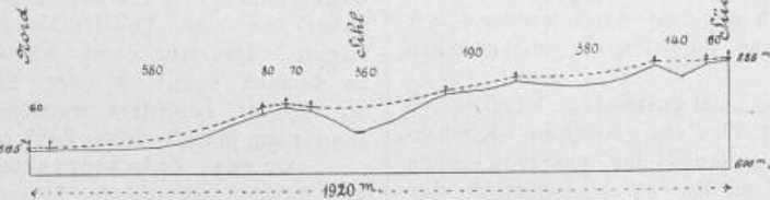
Fig. 2. Längenprofil. 1:20 000.
