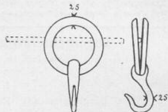
Fig. 6. Klemmring mit Haken. 1:10.
