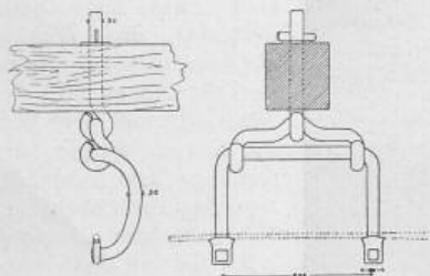
Fig. 4. Haken für Haupt- und Nebenseil. 1:30.
