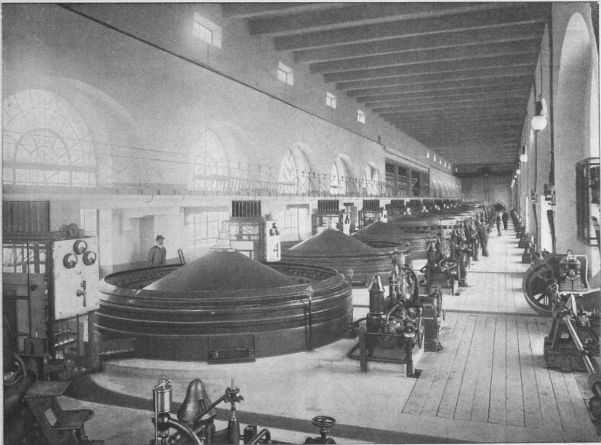
Fig. 10. Ansicht des Maschinenraumes. — Neue Gruppe.
