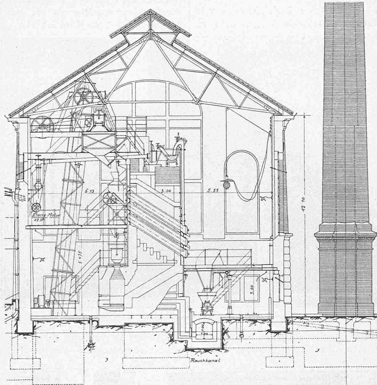
Fig. 12. Querschnitt A-B. Detail aus Tafel III. Masstab 1:200.
