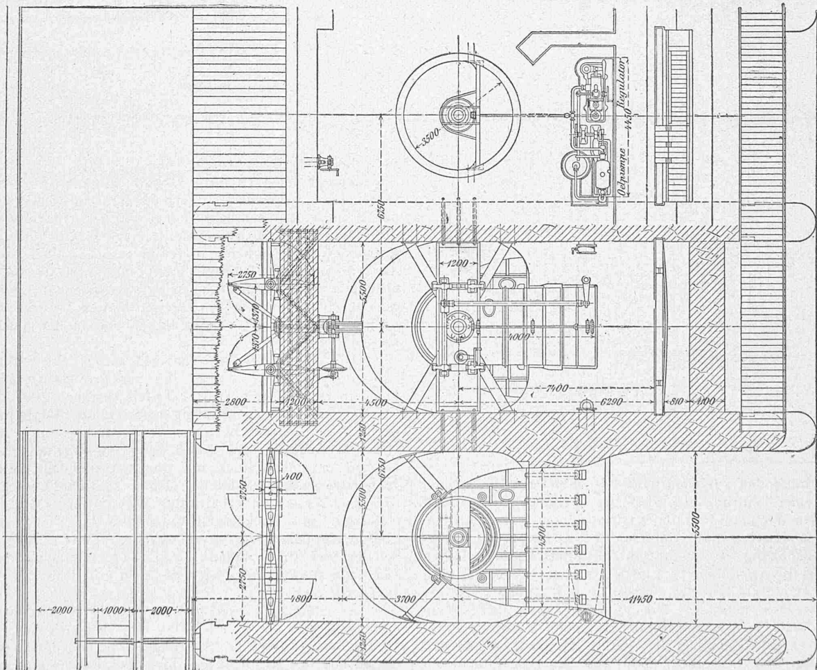
Fig. 3. Grundrisse 1:150.
