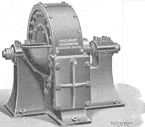
Schlagkreuzmühle.
