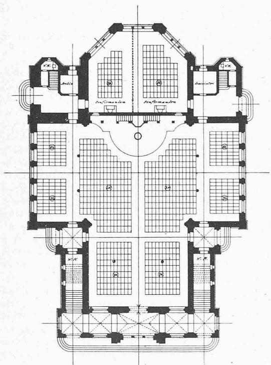
Erdgeschoss-Grundriss.
