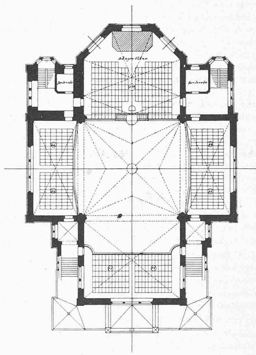
Emporen-Grundriss.
