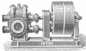
Hochdruckturbine mit direkt gekuppelter Gleichstromdynamo.
