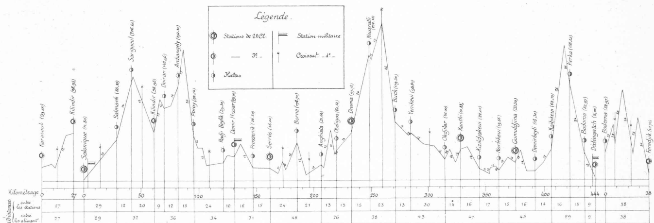
Profil en long. — Echelle 1 mm = 2,85 km, pour les hauteurs 1 mm = 6,7 m.
