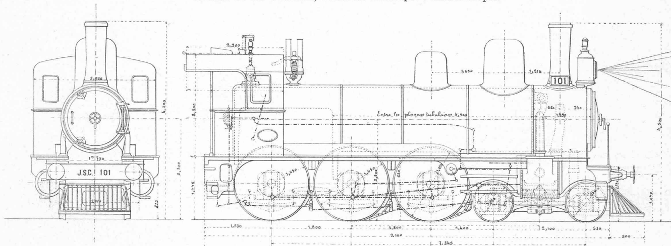
Chemin de fer Ottoman, Jonction Salonique-Constantinople.
